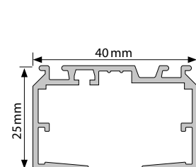
Querschnitt Profil
