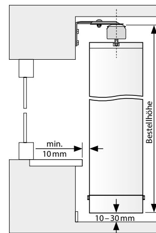
Montage mit Wandhalter
