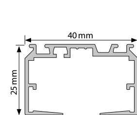
Querschnitt Profil
