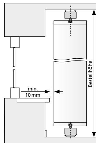
Montage verspannte Anlage/ Plafondanlage
