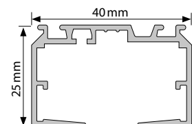
Querschnitt Profil
