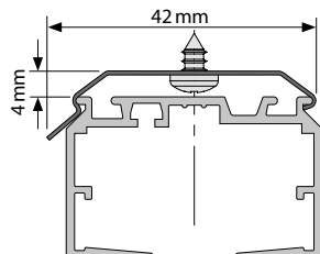
Querschnitt mit Standard-Clip
