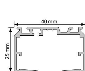
Querschnitt Profil
